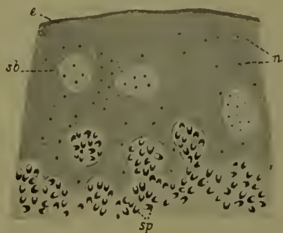
Fig. 54. Stück eines Schnittes durch die Hornhaut eines Stichelings, infiziert mit Nos. anomalum .
